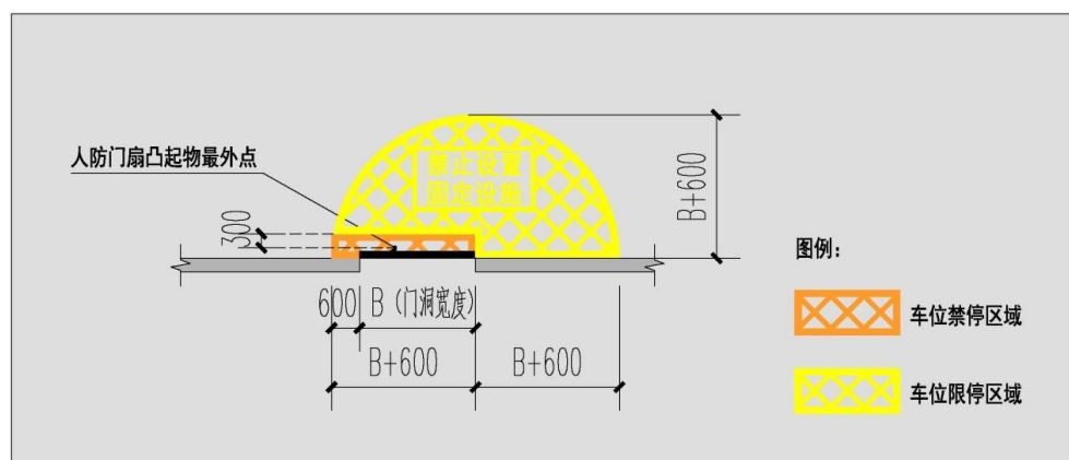
图 15 禁止与限制区域标识 4 (人防门平时常闭, 绞页在右侧)
