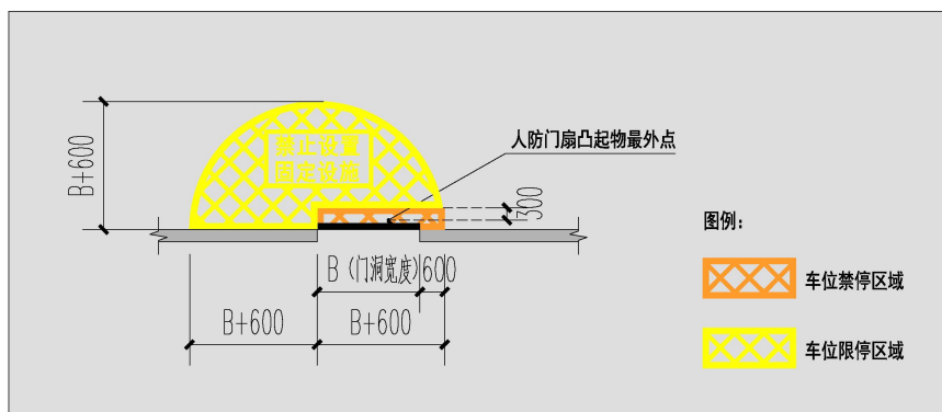
图 16 禁止与限制区域标识 5（人防门平时常闭，绞页在左侧）
