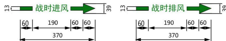
图 27 通风类管线标识样式及尺寸示例
