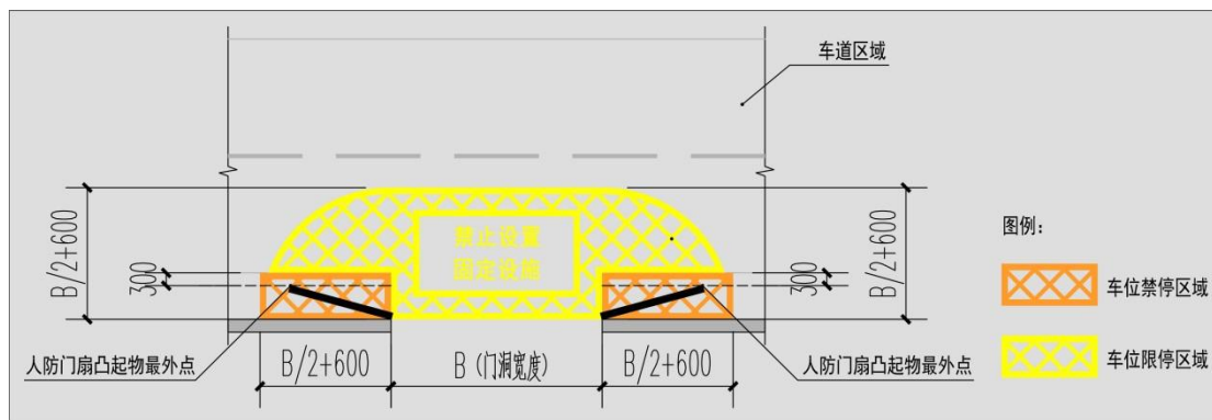
图 13 禁止与限制区域标识 2
