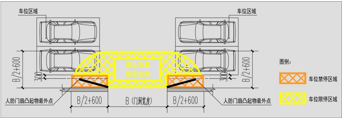
图12 禁止与限制区域标识1
