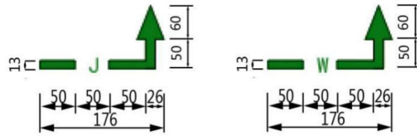
图 28 给水排水类管线标识样式及尺寸示例
